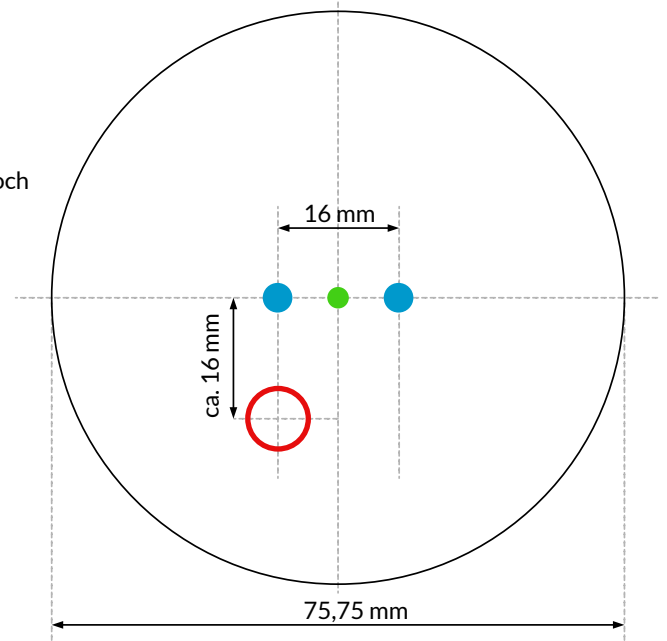
Bohrschablone iSHearo
